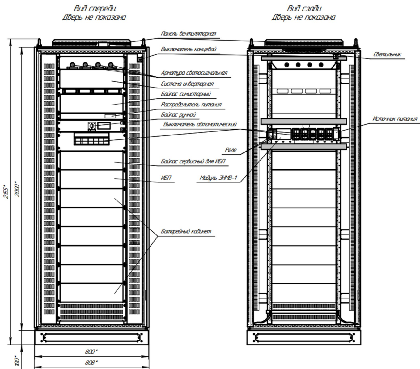
Рисунок 1. Общий вид и размеры шкафа № ЗНИ
