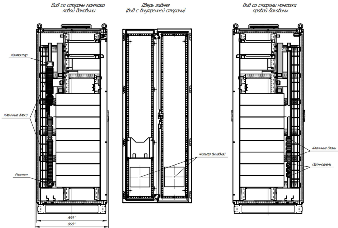
Рисунок 2. Общий вид шкафа № ЗНИ
